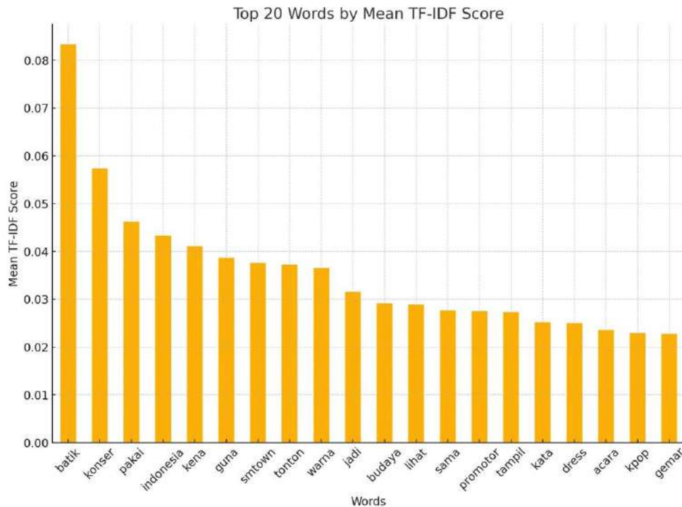
Gambar 7. 20 Kata dengan Nilai Rata-Rata TF-IDF Tertinggi
